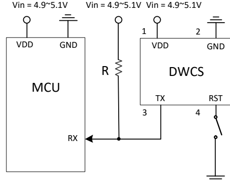
應用 2. MCU 接線 (UART:連續版別)
