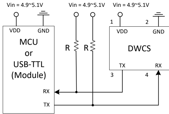
應用 1. MCU 或 USB-TTL 接線 (UART: AT 指令版別)
