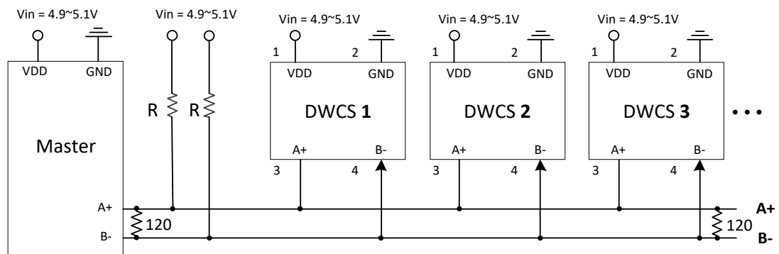
應用 5. RS485 接線
