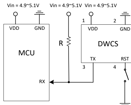
應用 2. MCU 接線 (UART:連續版別)
